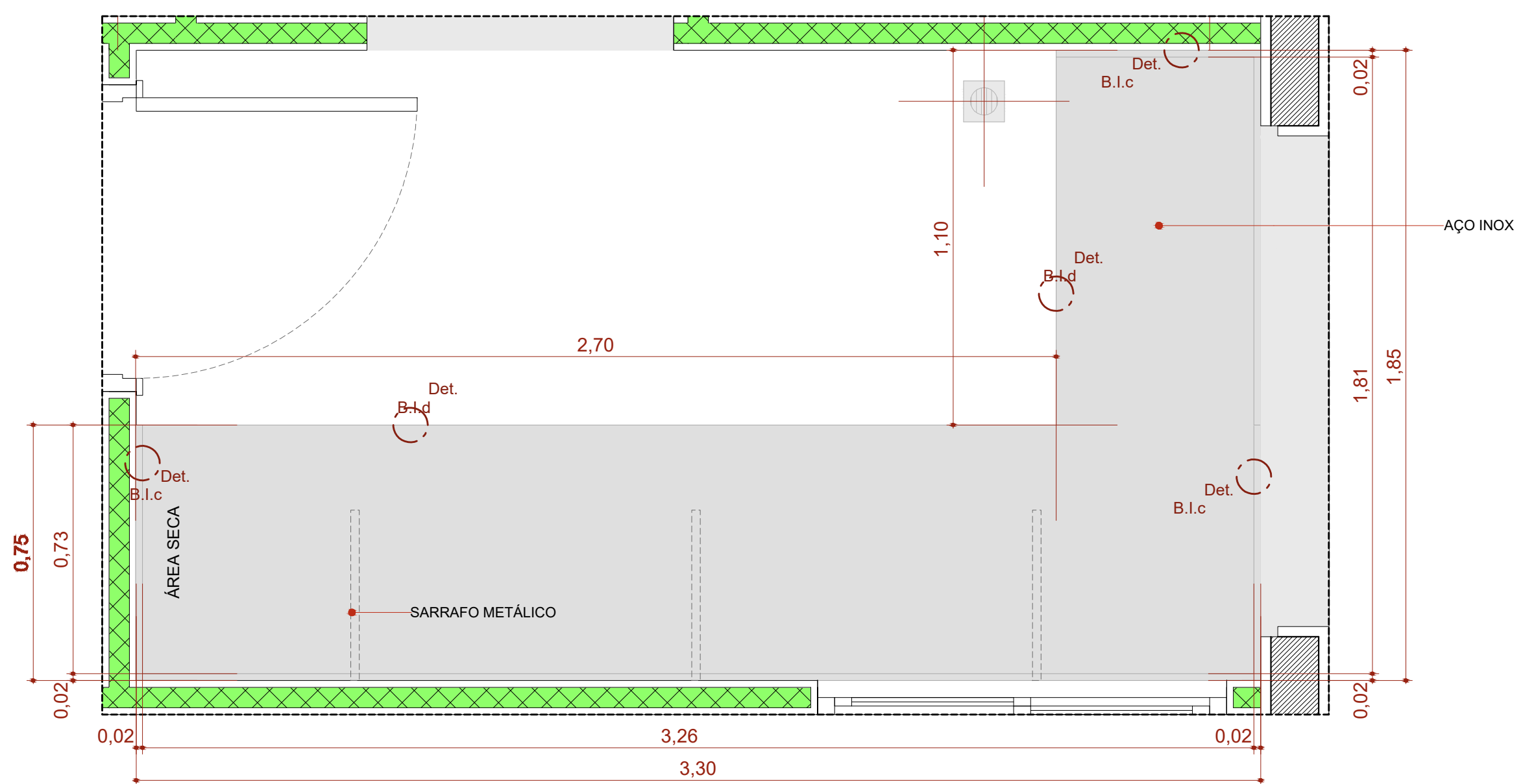
BI.330de Escala:1:20
