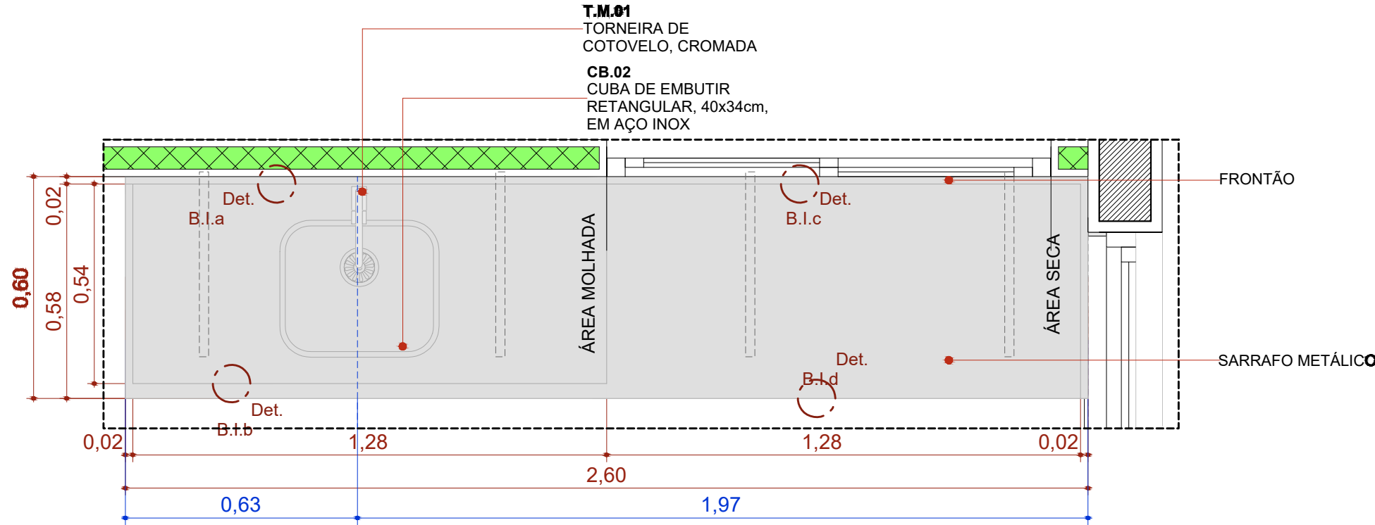
BIC.260d Escala:1:20
