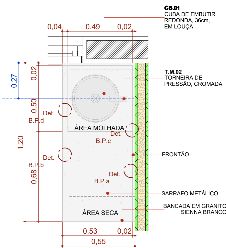
BPC.120e Escala:1:20
