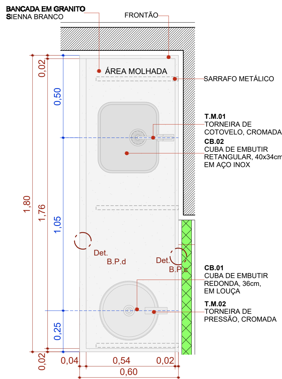
BPC.180e Escala:1:20
