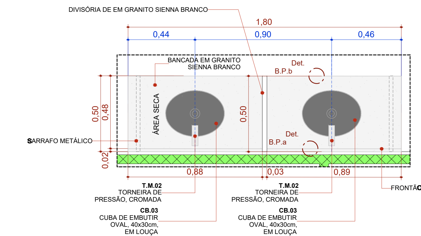
BPC.180-Escovário Escala:1:20
