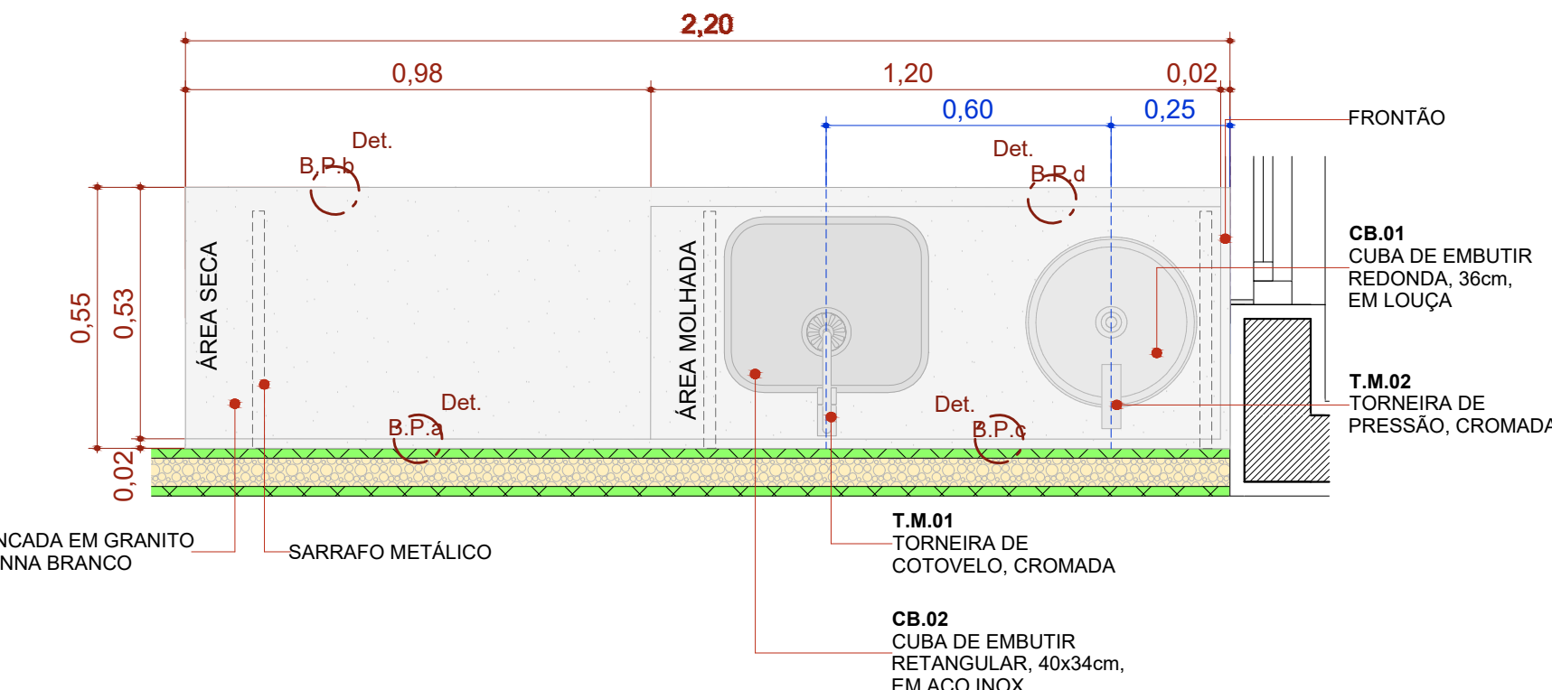
BPC.220e Escala:1:20
