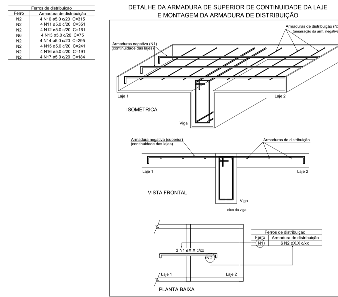
Armação negativa das lajes do pavimento TERREO (Eixo Y)
